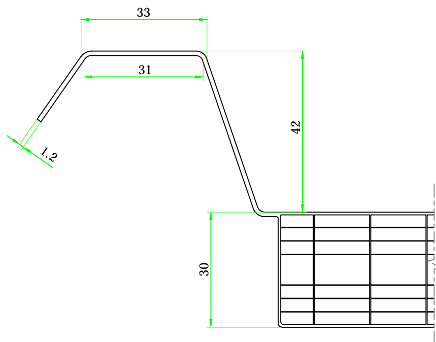
DETALLE LADO A ESCALA 1:1
