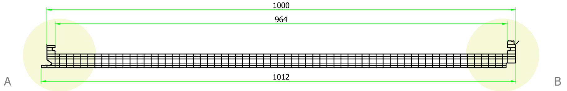
DETALLE GEOMETRÍA COMPLETA ESCALA 1:5
