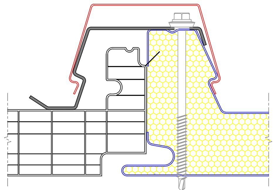
DETALLE DE ENCAJE CON PANEL DE POLIURETANO DE 30mm ESCALA 1:1
