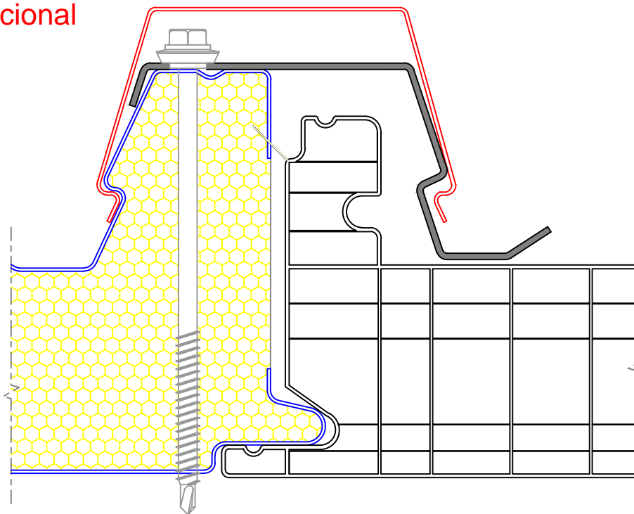
DETALLE LADO A ESCALA 1:1
