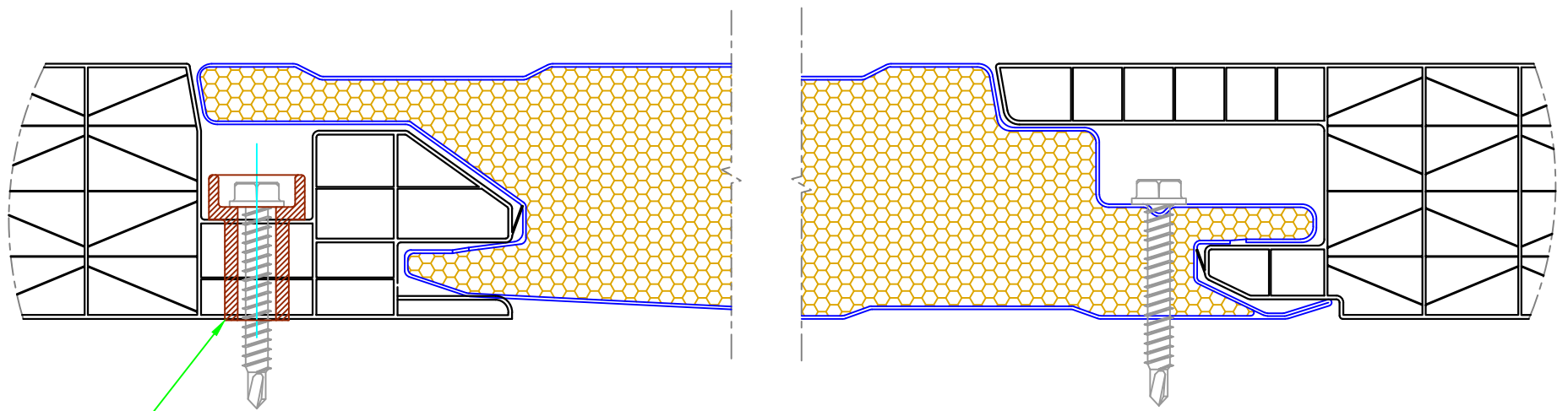
DETALLE ENCUENTRO CON ITALPANNELLI FACHADA ESCALA 1:1
