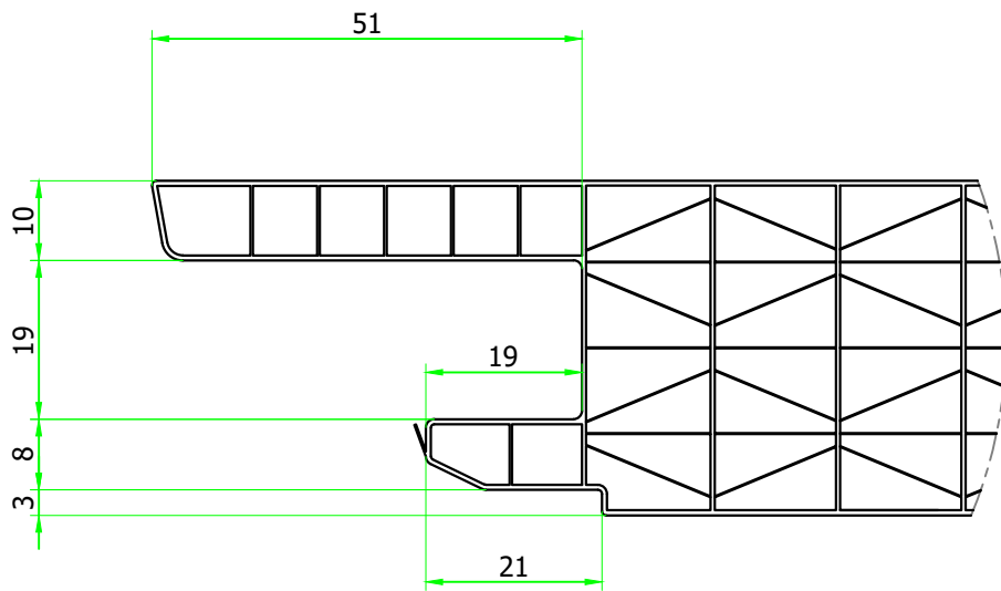
DETALLE LADO A ESCALA 1:1
