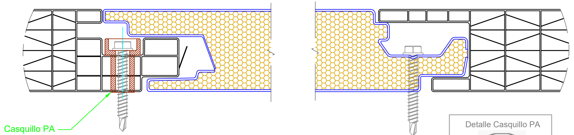
DETALLE ENCUENTRO CON PERFIMUR ESCALA 1:1
