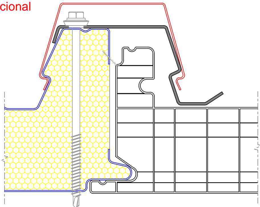
DETALLE DE ENCAJE CON PANEL DE POLIURETANO DE 40mm ESCALA 1:1
