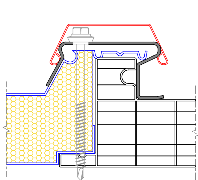
DETALLE DE ENCAJE CON PANEL DE POLIURETANO DE 30mm ESCALA 1:1
