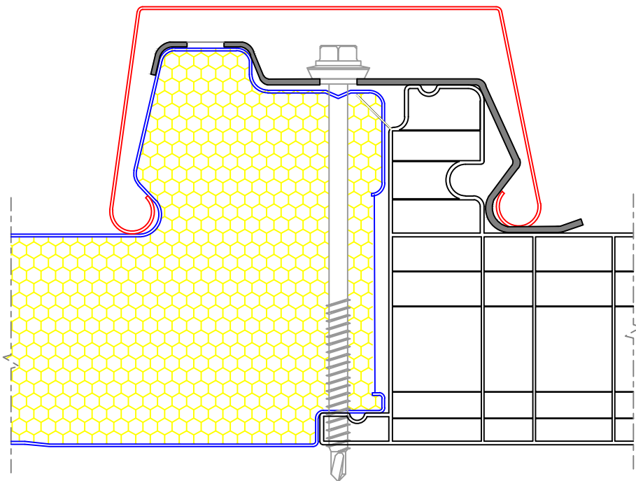
DETALLE DE ENCAJE CON PANEL DE POLIURETANO DE 30mm ESCALA 1:1
