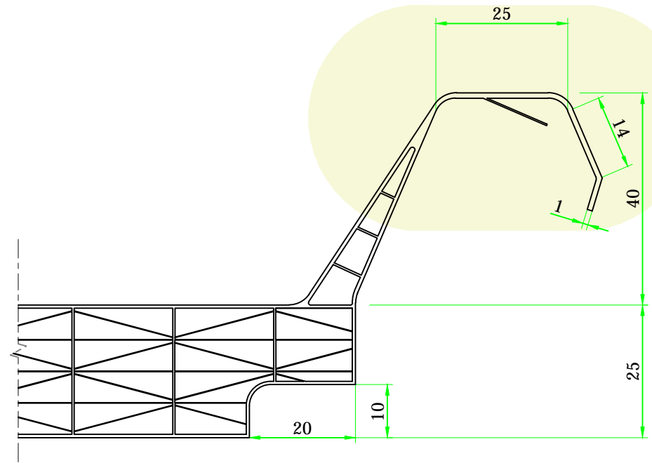
DETALLE LADO B ESCALA 1:1
