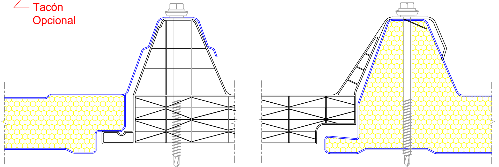
DETALLE DE ENCAJE CON PANEL DE POLIURETANO DE 30mm ESCALA 1:1
