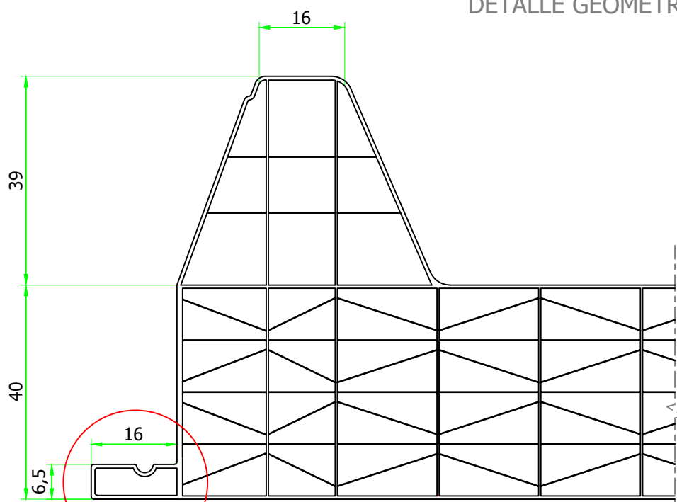
DETALLE LADO A ESCALA 1:1
