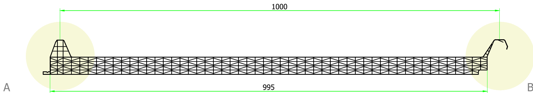
DETALLE GEOMETRÍA COMPLETA ESCALA 1:5
